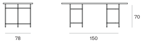
E3 390×78 mittig
