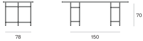
E3 290×78 mittig
